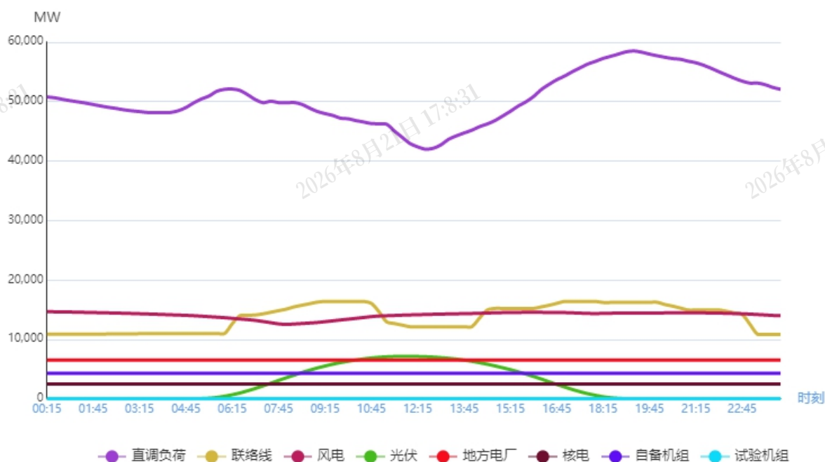
图 1 5月5日负荷及电源出力预测情况
