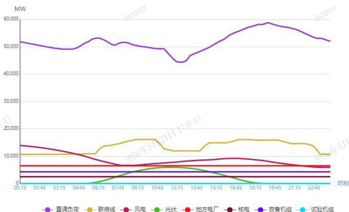
图1 5月6日负荷及电源出力预测情况
