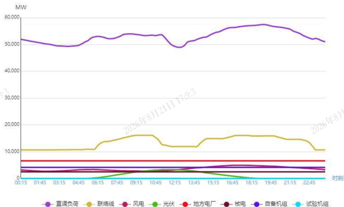
图1 5月8日负荷及电源出力预测情况
