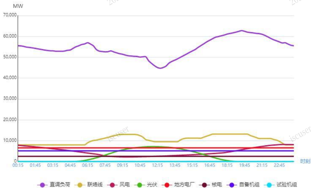
图1 5月20日负荷及电源出力预测情况
