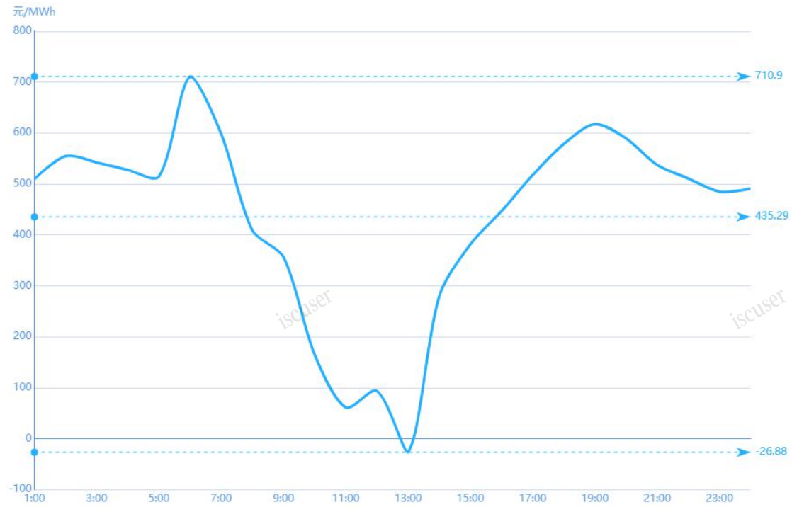
图4 5月20日实时市场用电侧价格
