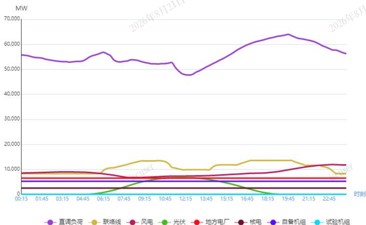
图 2 5 月 24 日负荷及电源出力预测情况
