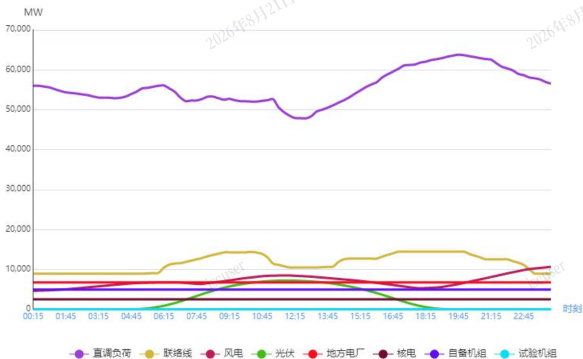
图1 5月26日负荷及电源出力预测情况
