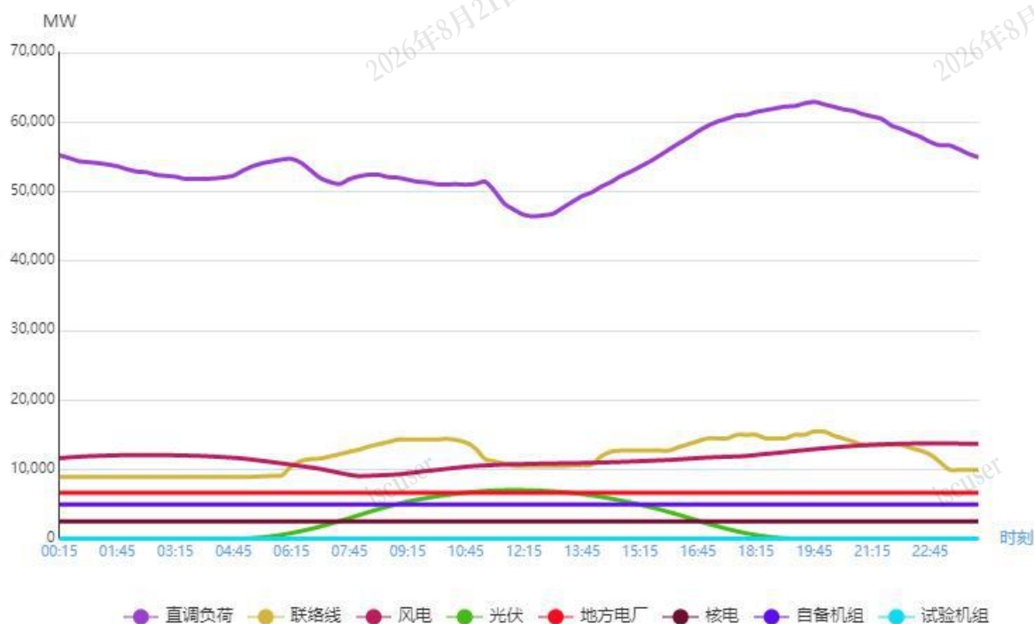
图1 5月28日负荷及电源出力预测情况
