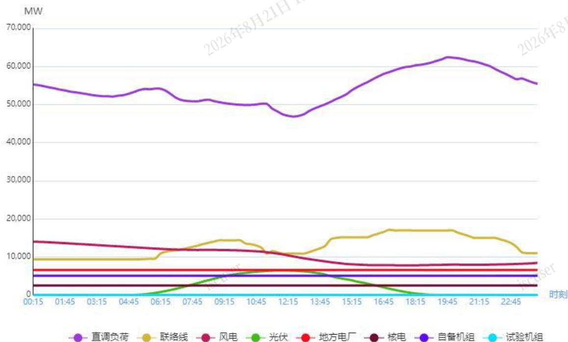
图 1 5 月 29 日负荷及电源出力预测情况
