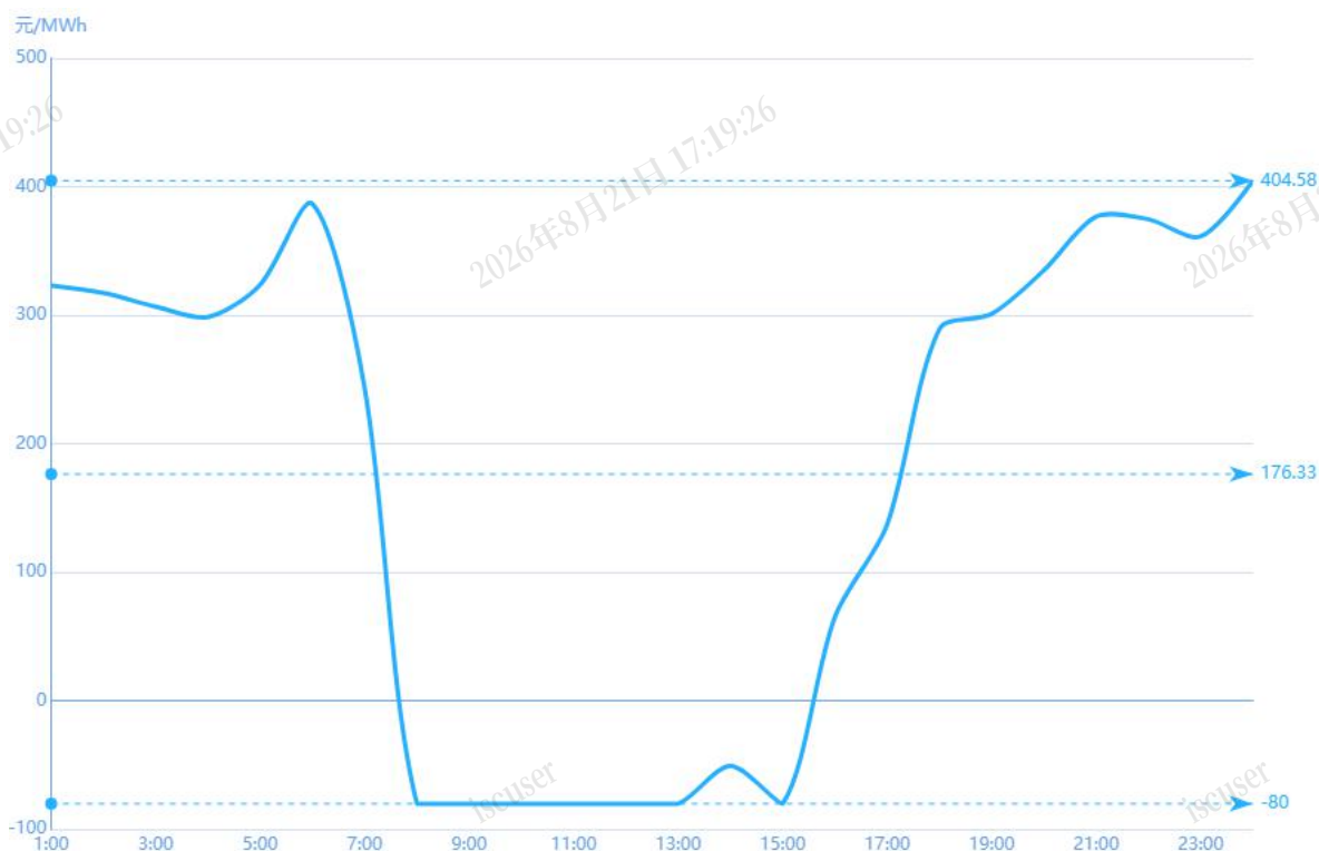
图 3 5 月 31 日实时市场用电侧价格
