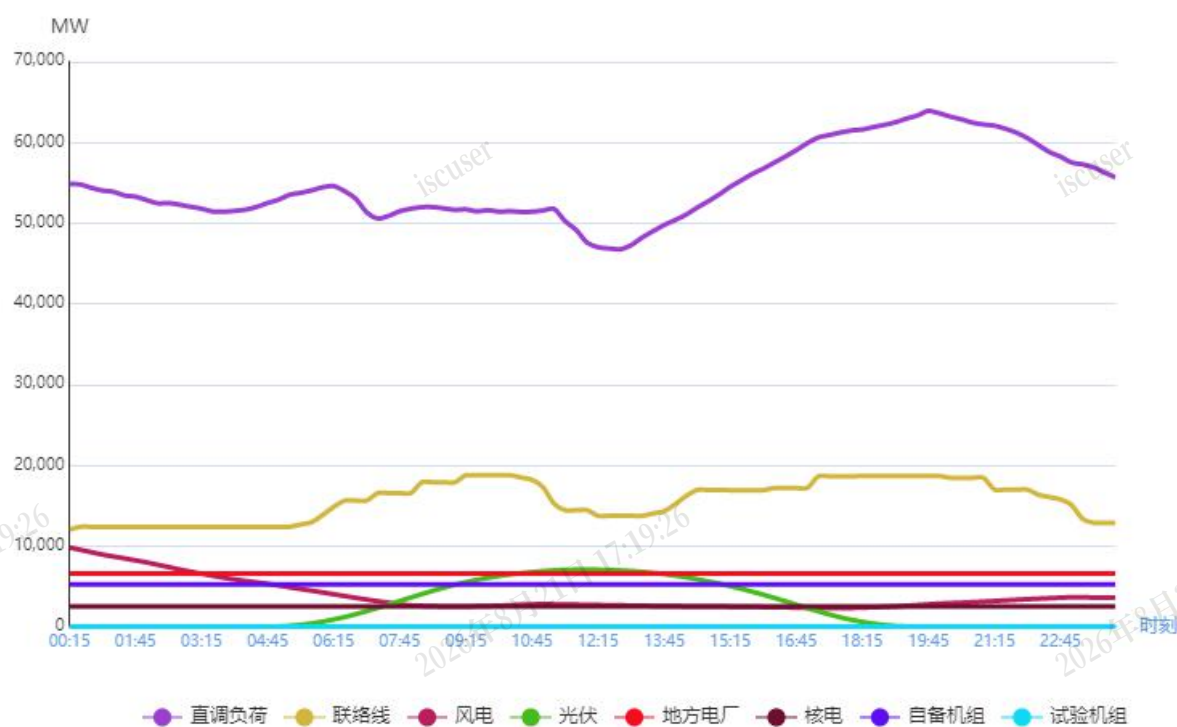
图1 6月1日负荷及电源出力预测情况
