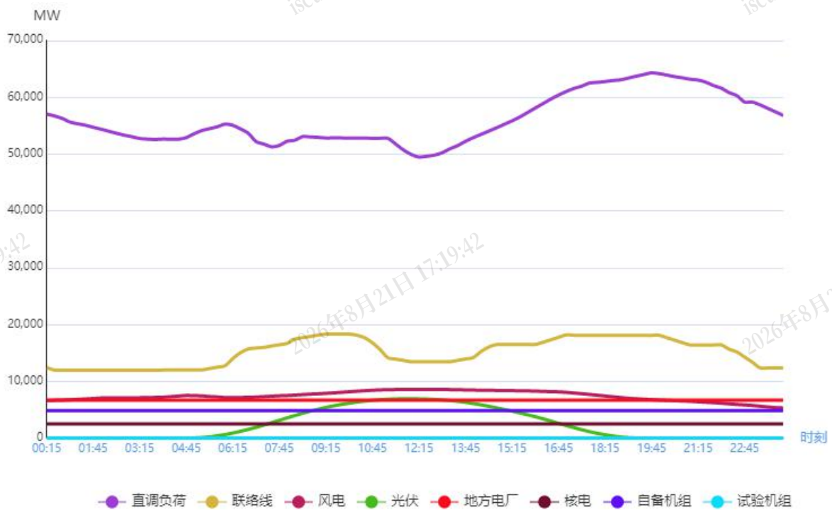
图2 6月6日负荷及电源出力预测情况
