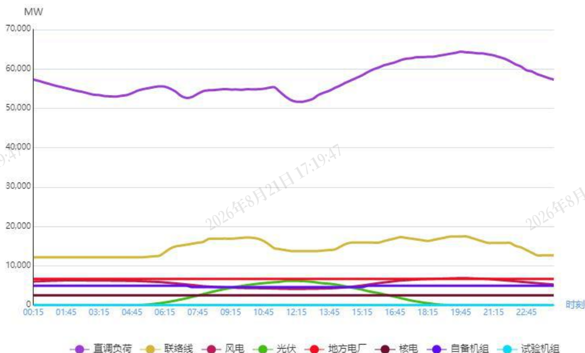
图1 6月8日负荷及电源出力预测情况
