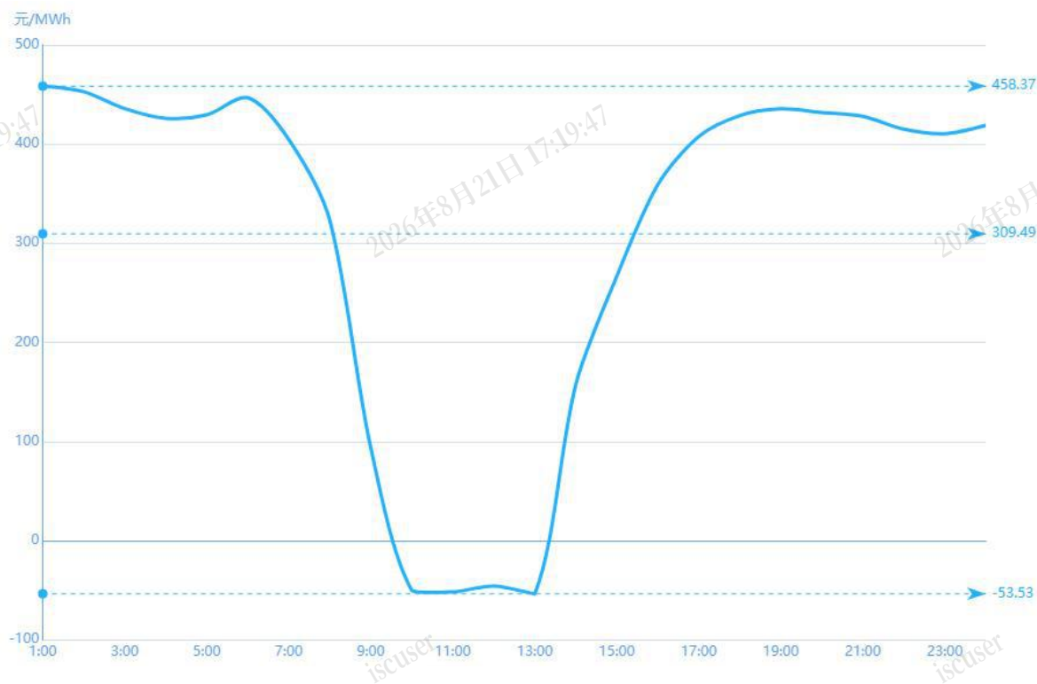
图 3 6 月 7 日实时市场用电侧价格
