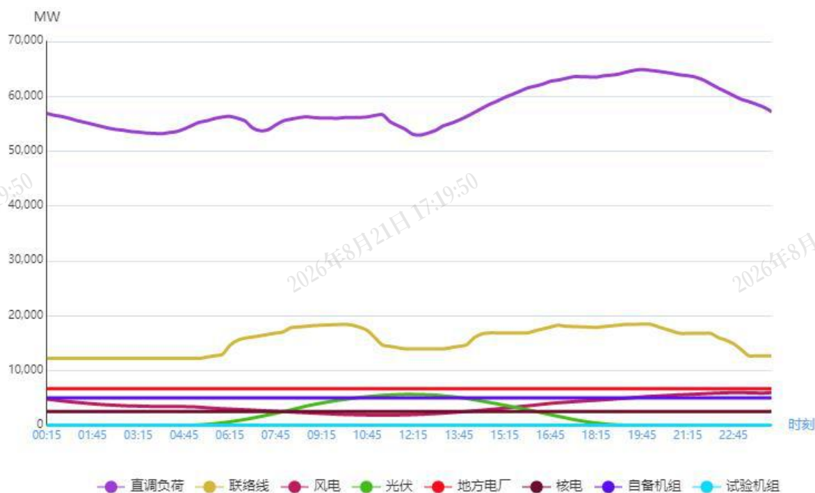
图1 6月9日负荷及电源出力预测情况
