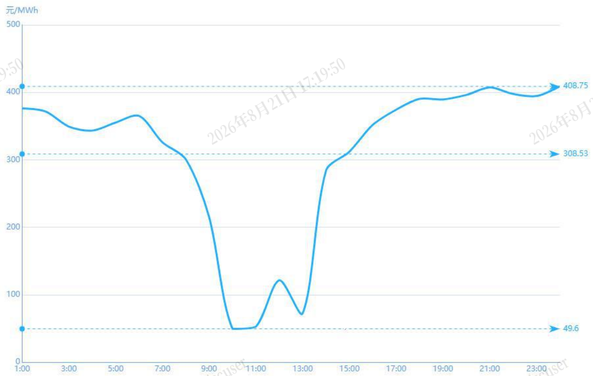
图 3 6 月 8 日实时市场用电侧价格
