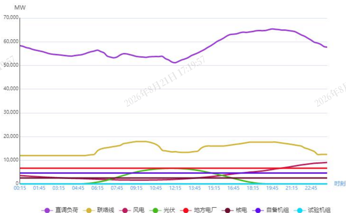
图2 6月11日负荷及电源出力预测情况
