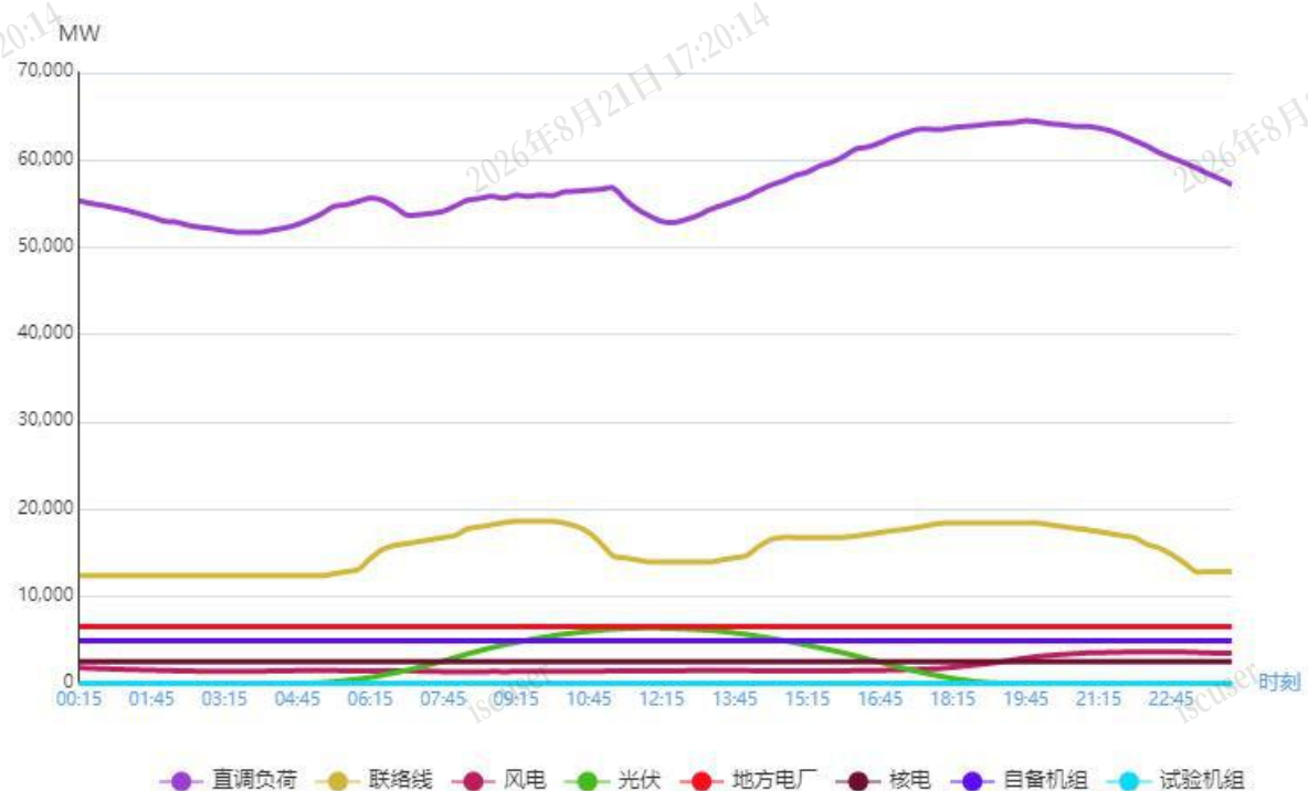
图1 6月15日负荷及电源出力预测情况
