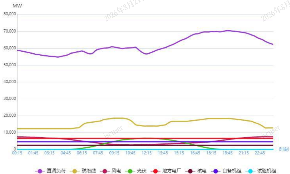
图2 6月17日负荷及电源出力预测情况
