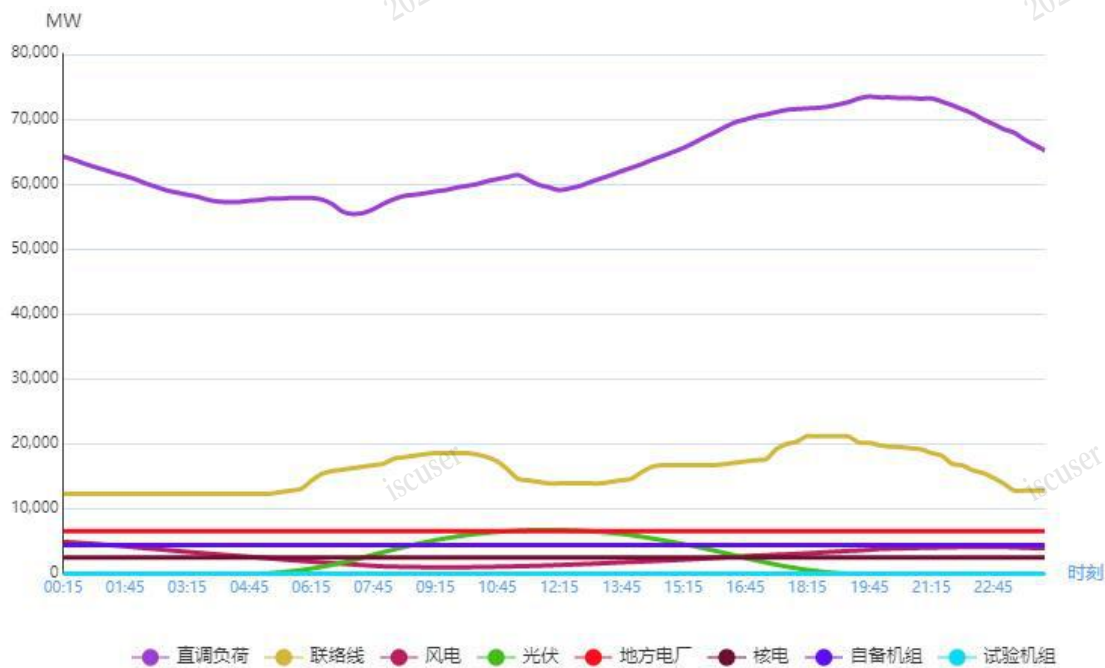
图1 6月19日负荷及电源出力预测情况
