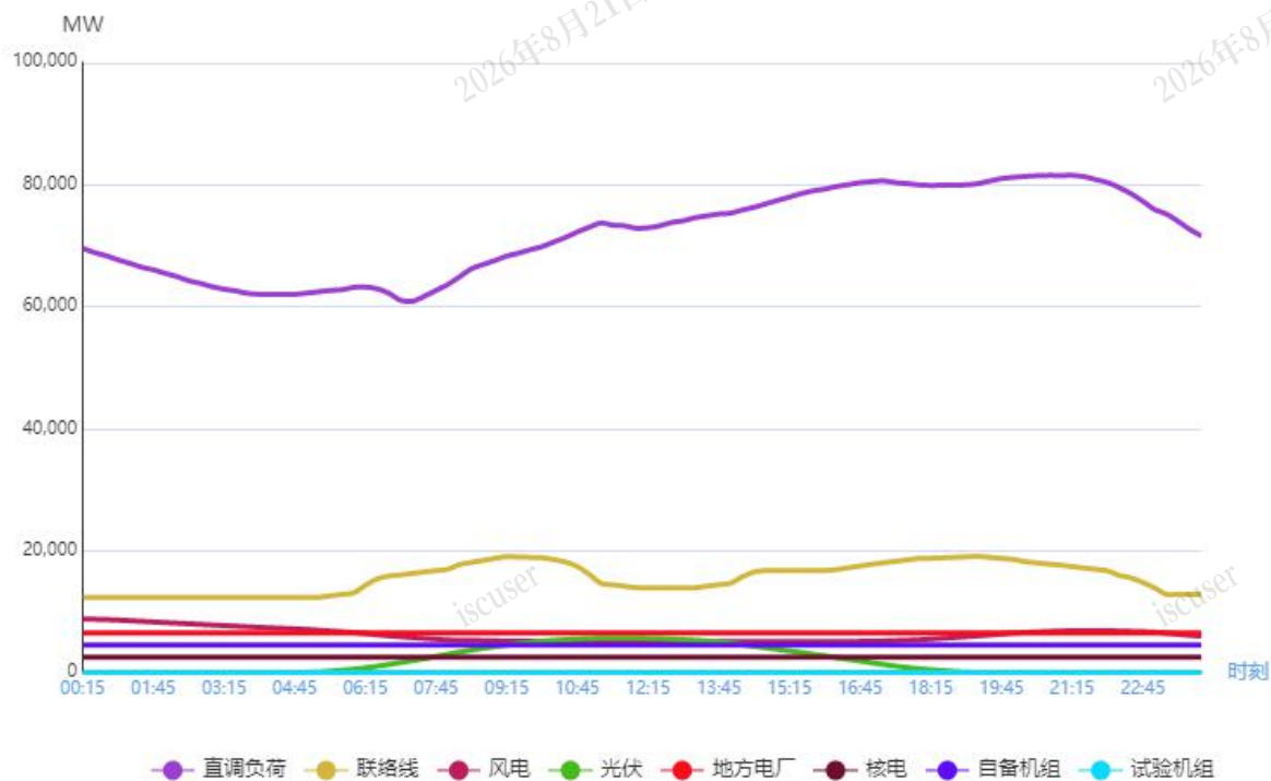
图2 6月22日负荷及电源出力预测情况
