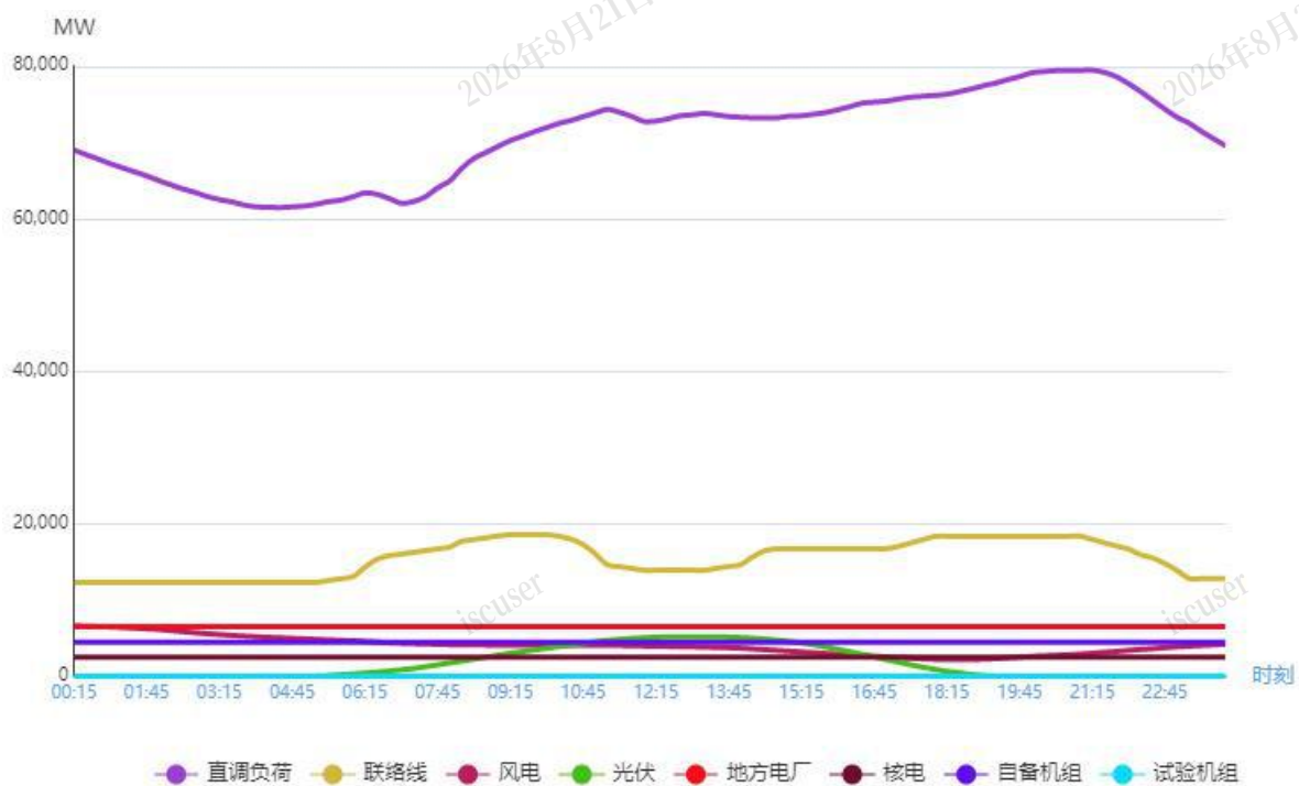
图1 6月23日负荷及电源出力预测情况
