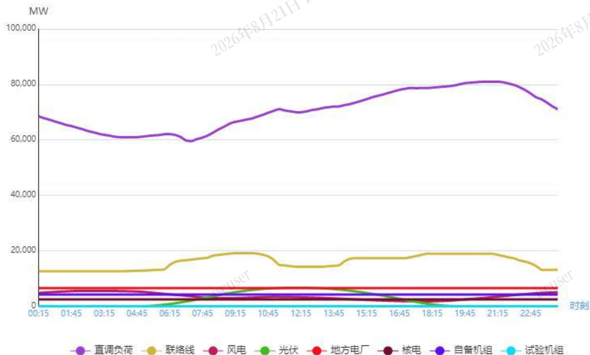
图 1 6 月 24 日负荷及电源出力预测情况
