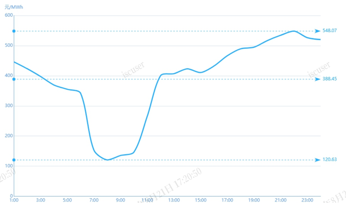
图3 6月25日实时市场用电侧价格
