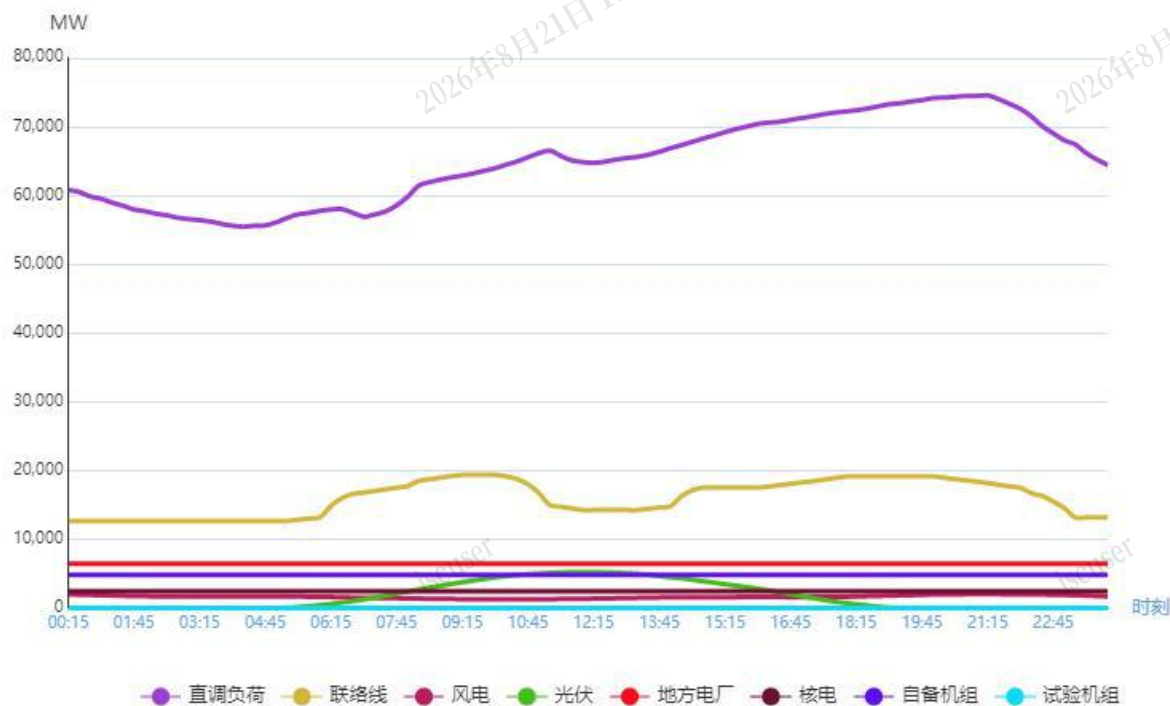
图 1 6 月 29 日负荷及电源出力预测情况
