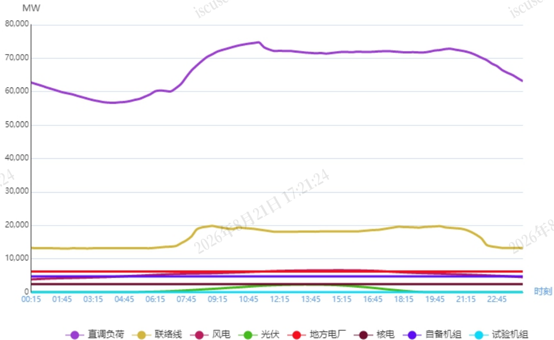
图1 7月6日负荷及电源出力预测情况
