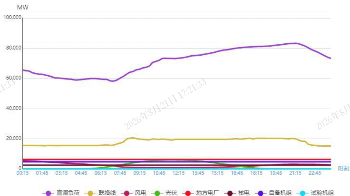
图1 7月9日负荷及电源出力预测情况
