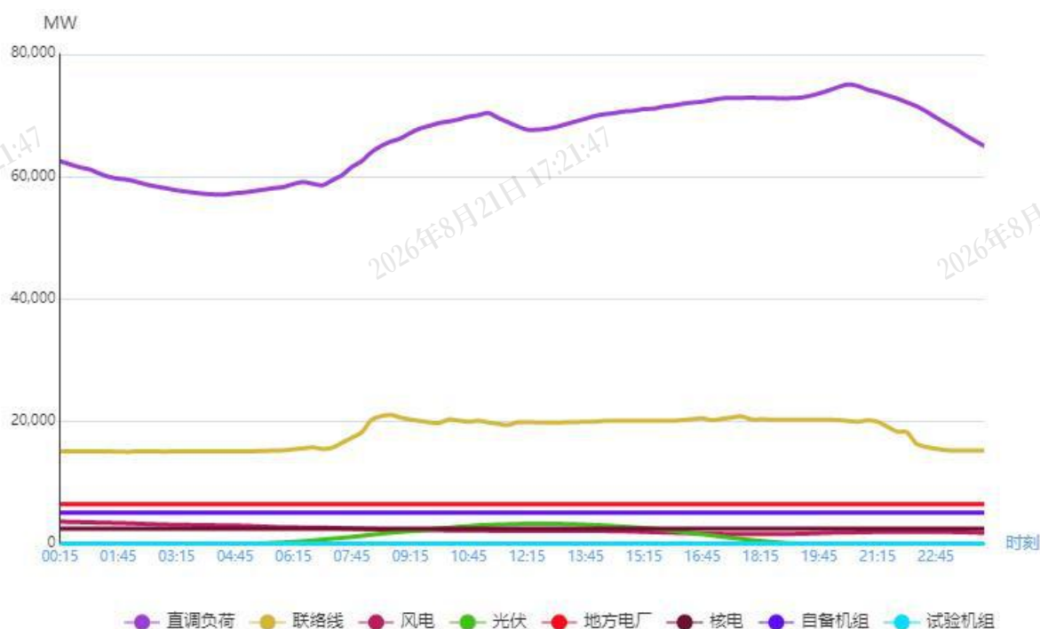
图1 7月13日负荷及电源出力预测情况
