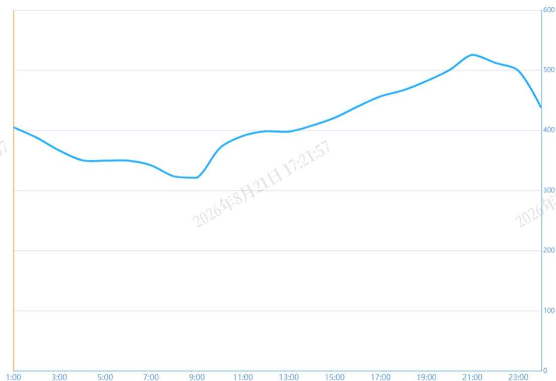
图 2 7 月 16 日日前市场用电侧价格
