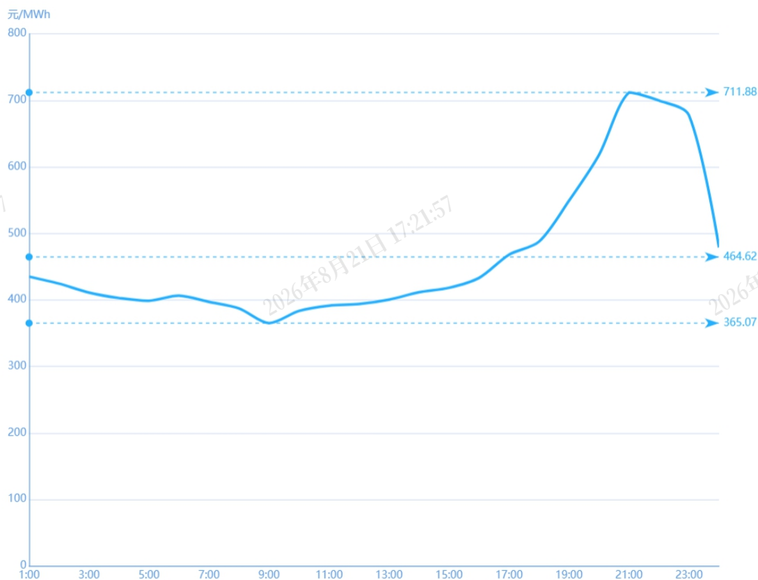
图 3 7 月 15 日实时市场用电侧价格
