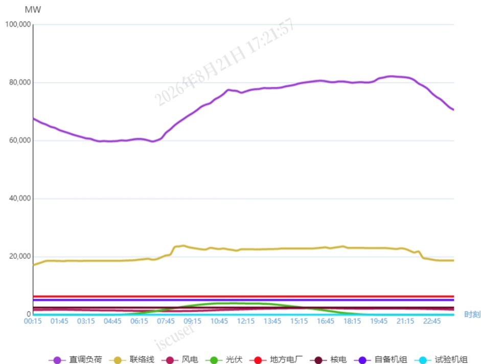
图1 7月16日负荷及电源出力预测情况
