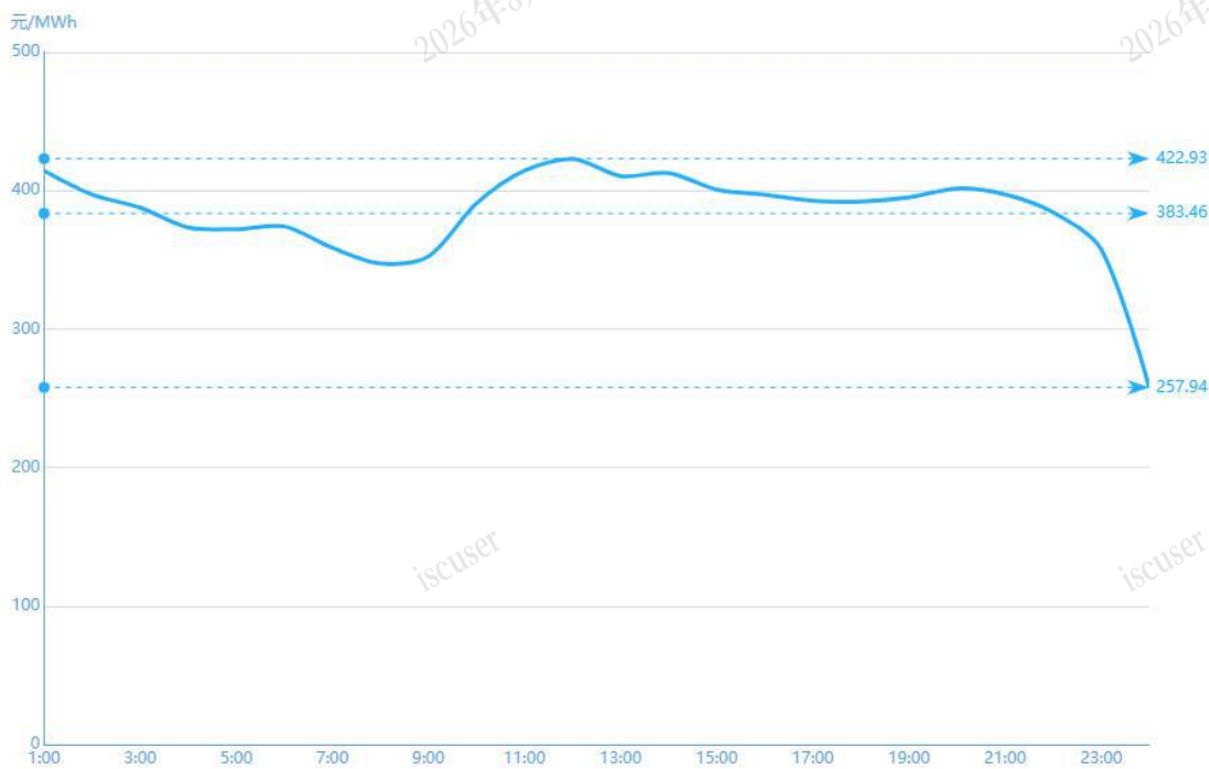
图 3 7 月 16 日实时市场用电侧价格
