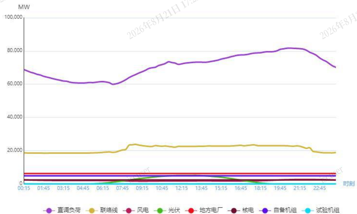
图1 7月17日负荷及电源出力预测情况
