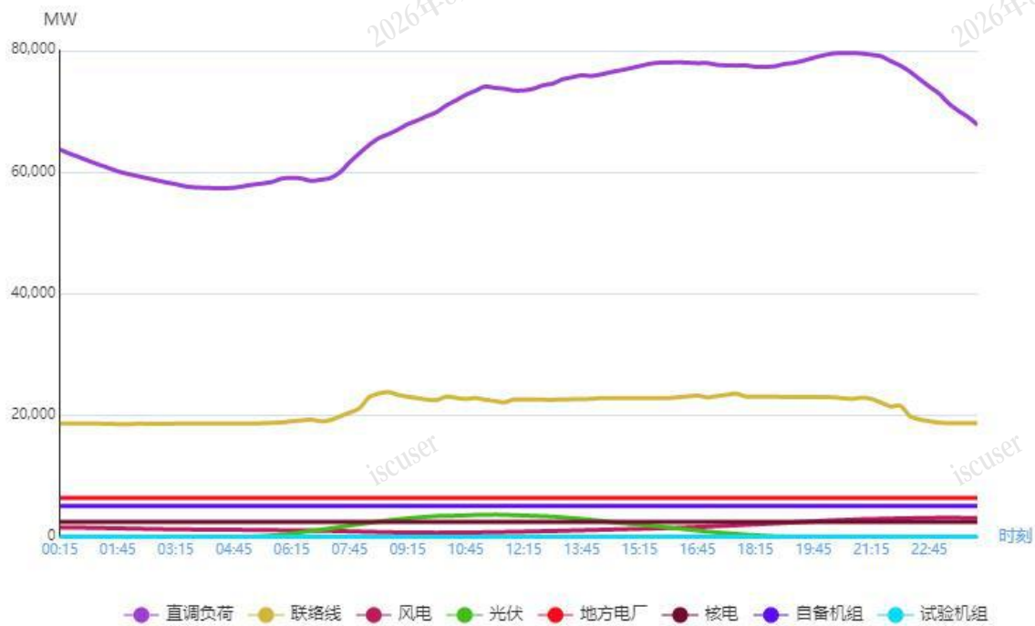
图1 7月19日负荷及电源出力预测情况
