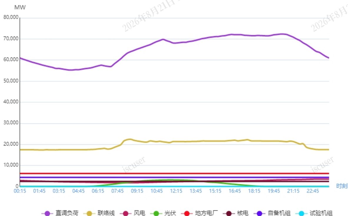
图 1 7 月 28 日负荷及电源出力预测情况
