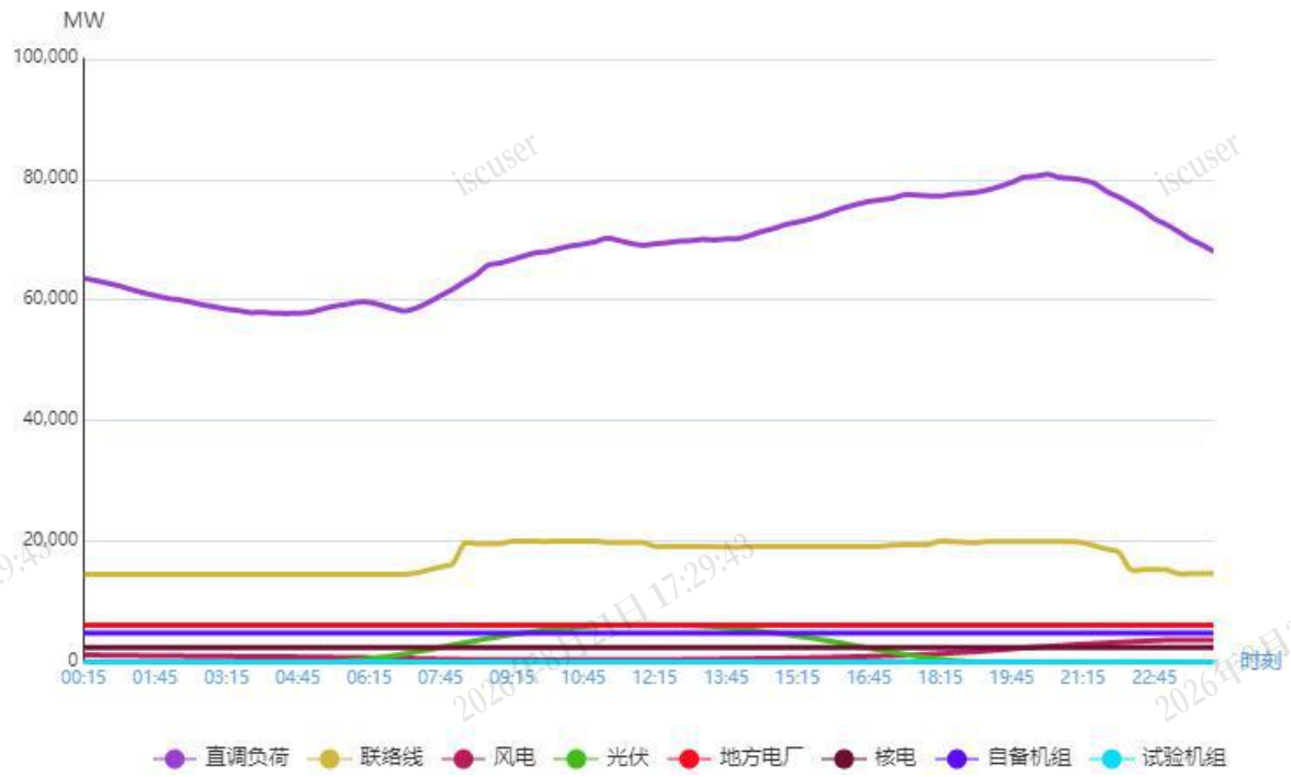
图 1 8月2日负荷及电源出力预测情况
