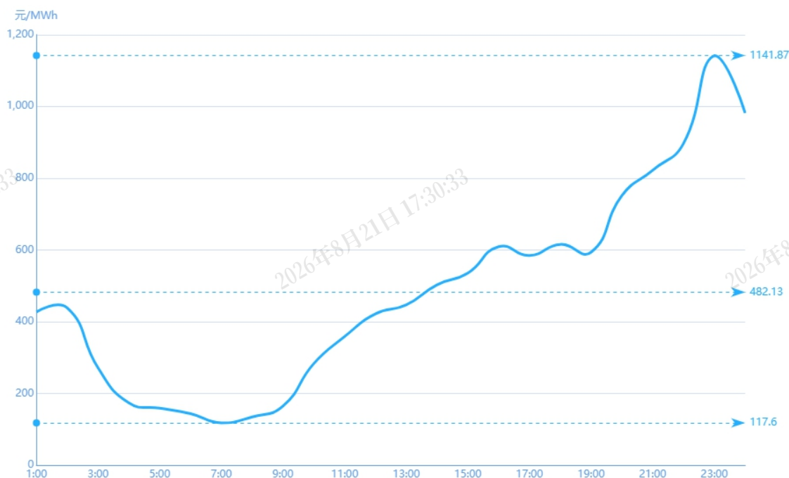
图 3 8 月 7 日实时市场用电侧价格
