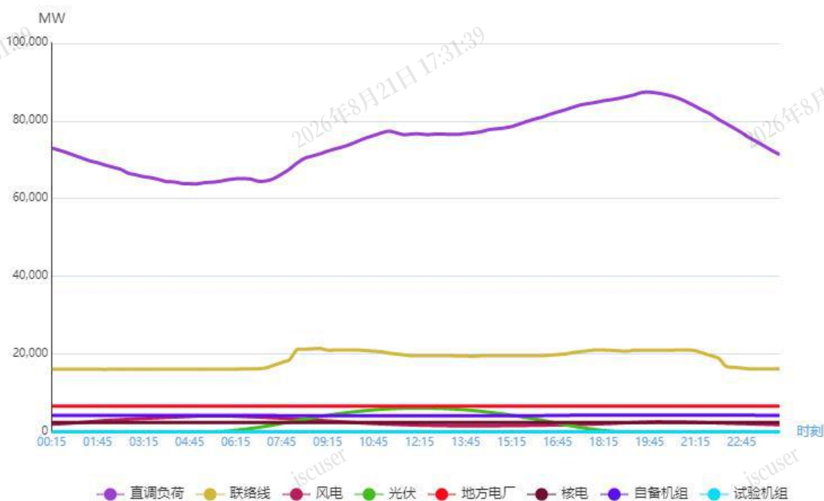
图1 8月16日负荷及电源出力预测情况
