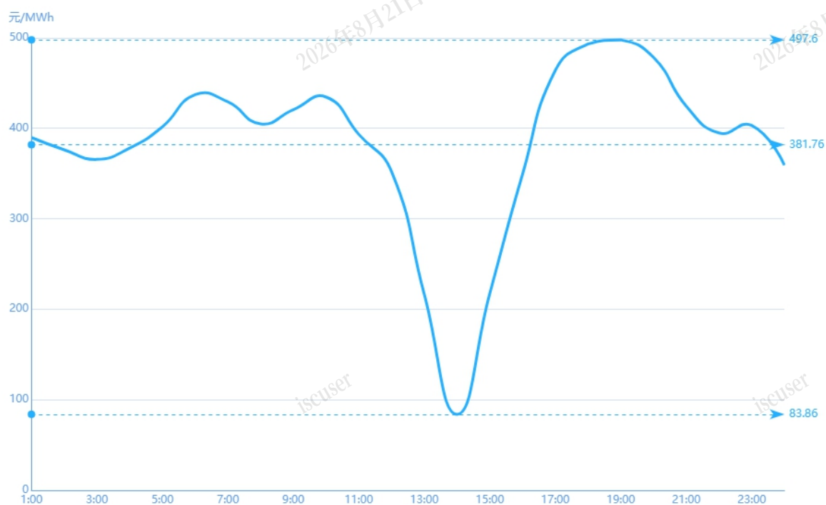
图3 8月25日实时市场用电侧价格
