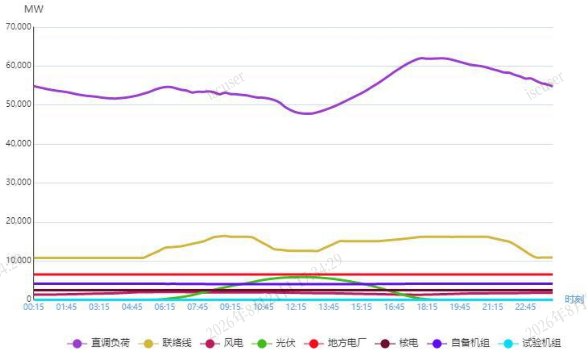
图 1 9月4日负荷及电源出力预测情况
