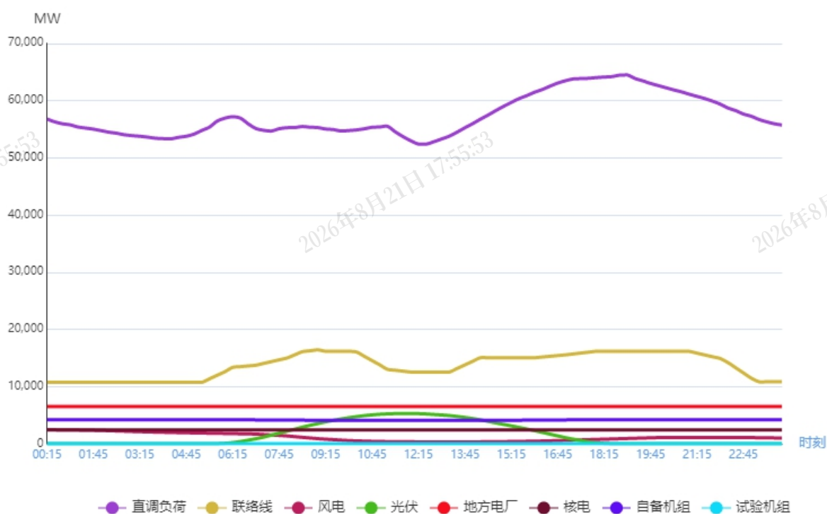
图1 9月9日负荷及电源出力预测情况
