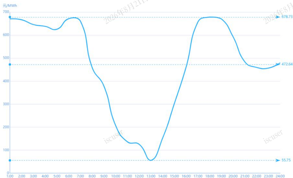
图3 9月28日实时市场用电侧价格
