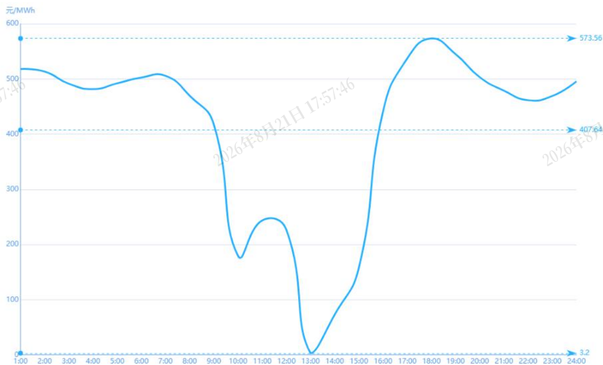
图 3 10 月 15 日实时市场用电侧价格
