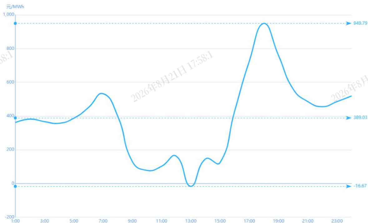
图 3 10 月 20 日实时市场用电侧价格
