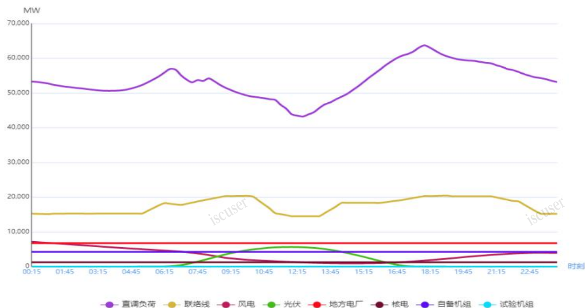
图1 10月21日负荷及电源出力预测情况
