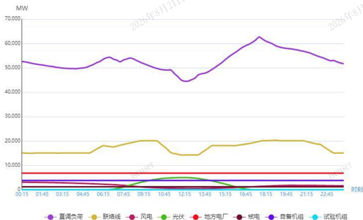
图 1 10 月 29 日负荷及电源出力预测情况
