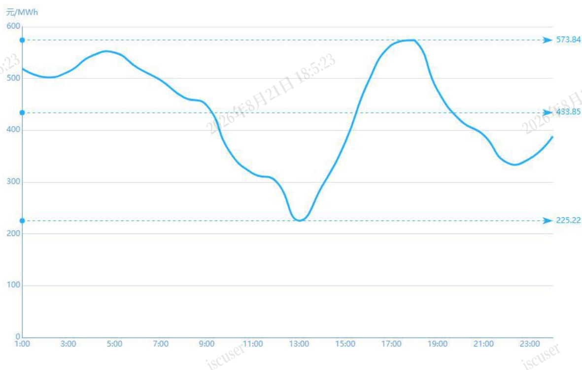
图 3 11 月 8 日实时市场用电侧价格
