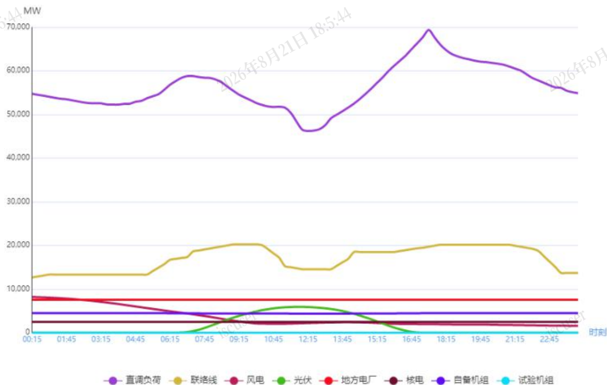
图1 11月15日负荷及电源出力预测情况
