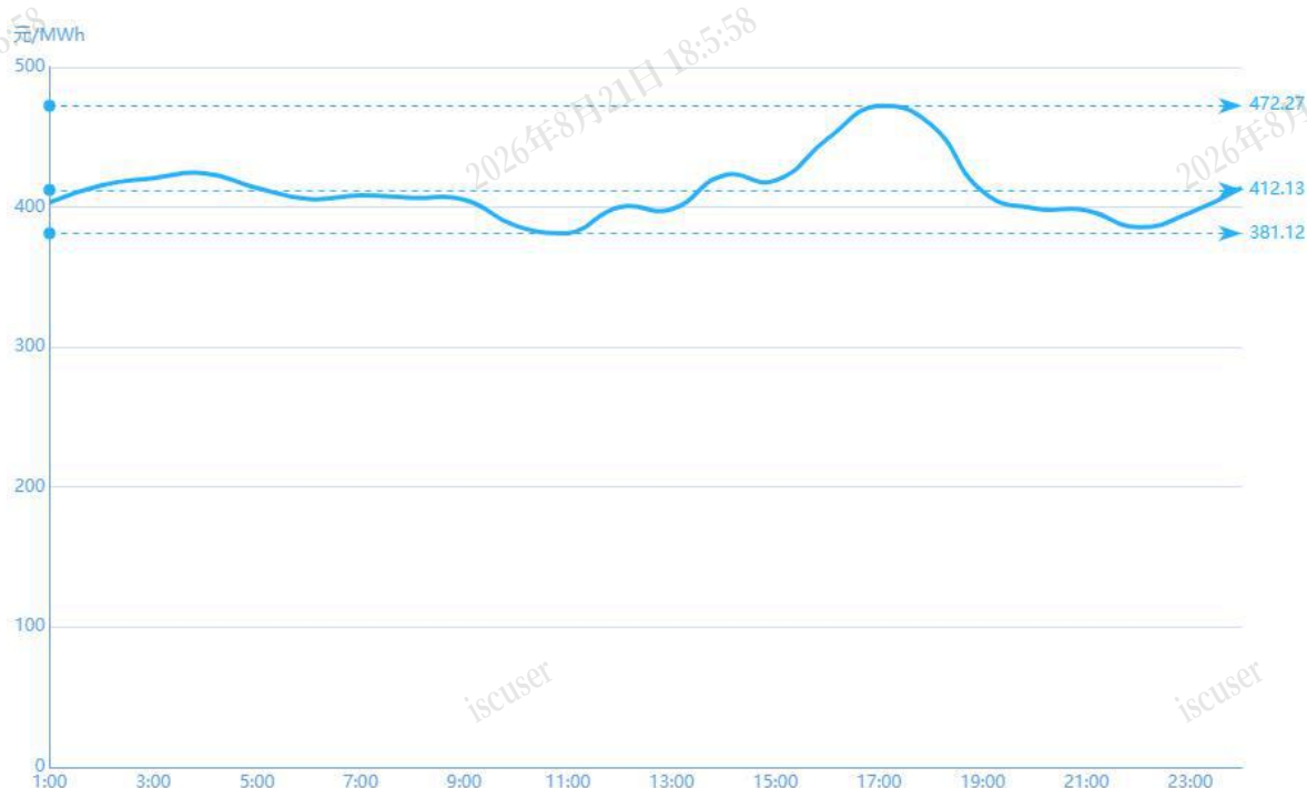
图 3 11 月 18 日实时市场用电侧价格
