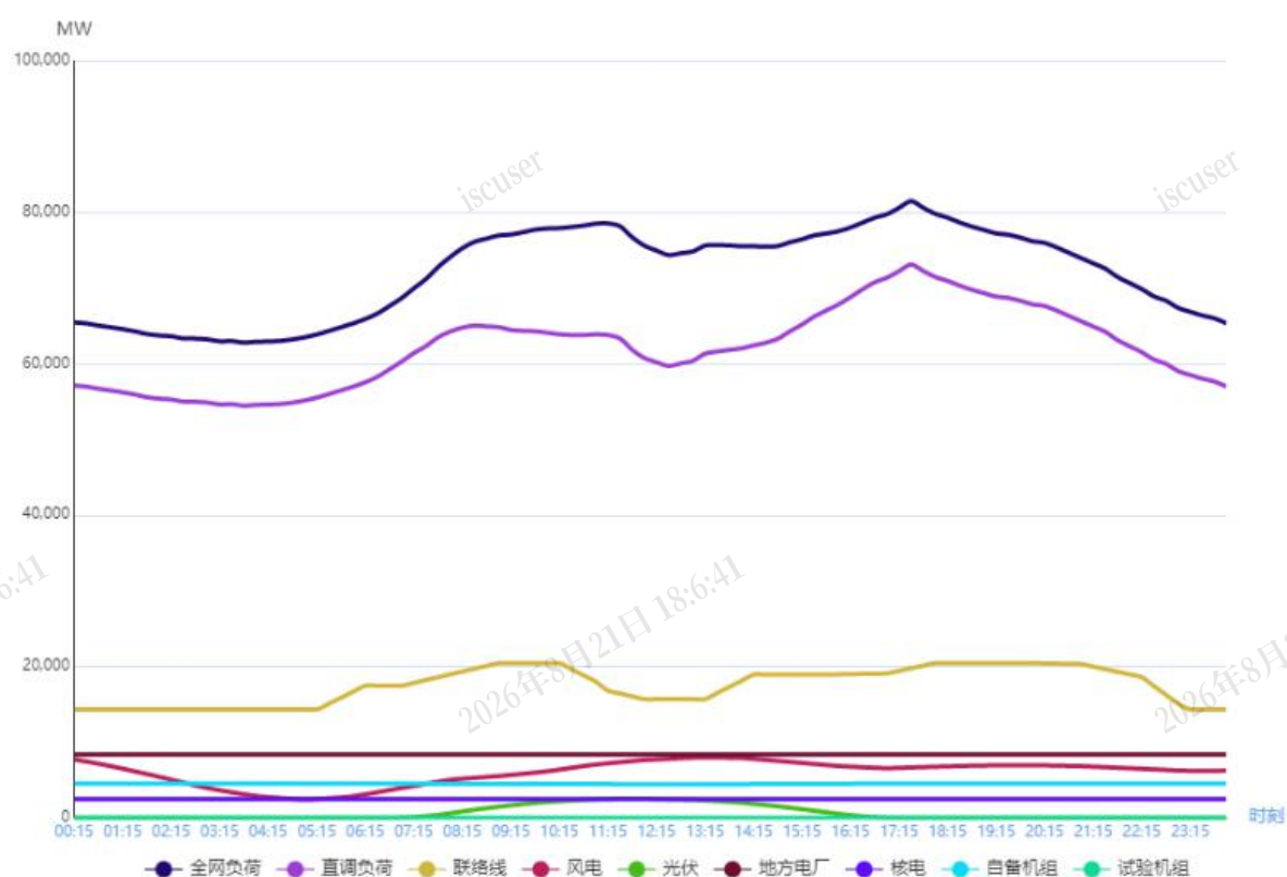
图1 12月3日负荷及电源出力预测情况
