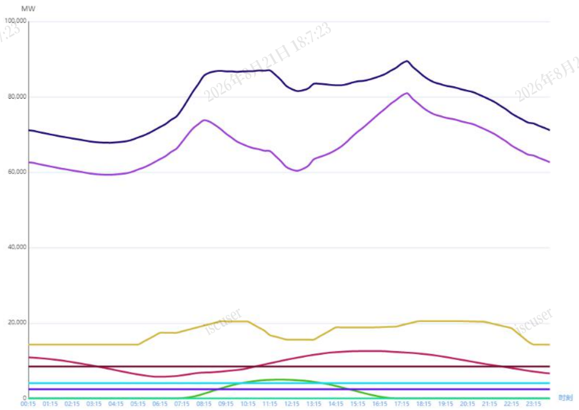
图1 12月15日负荷及电源出力预测情况
