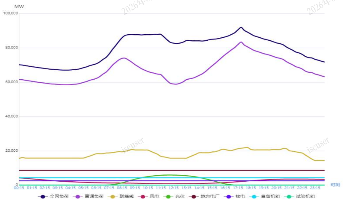
图1 12月19日负荷及电源出力预测情况
