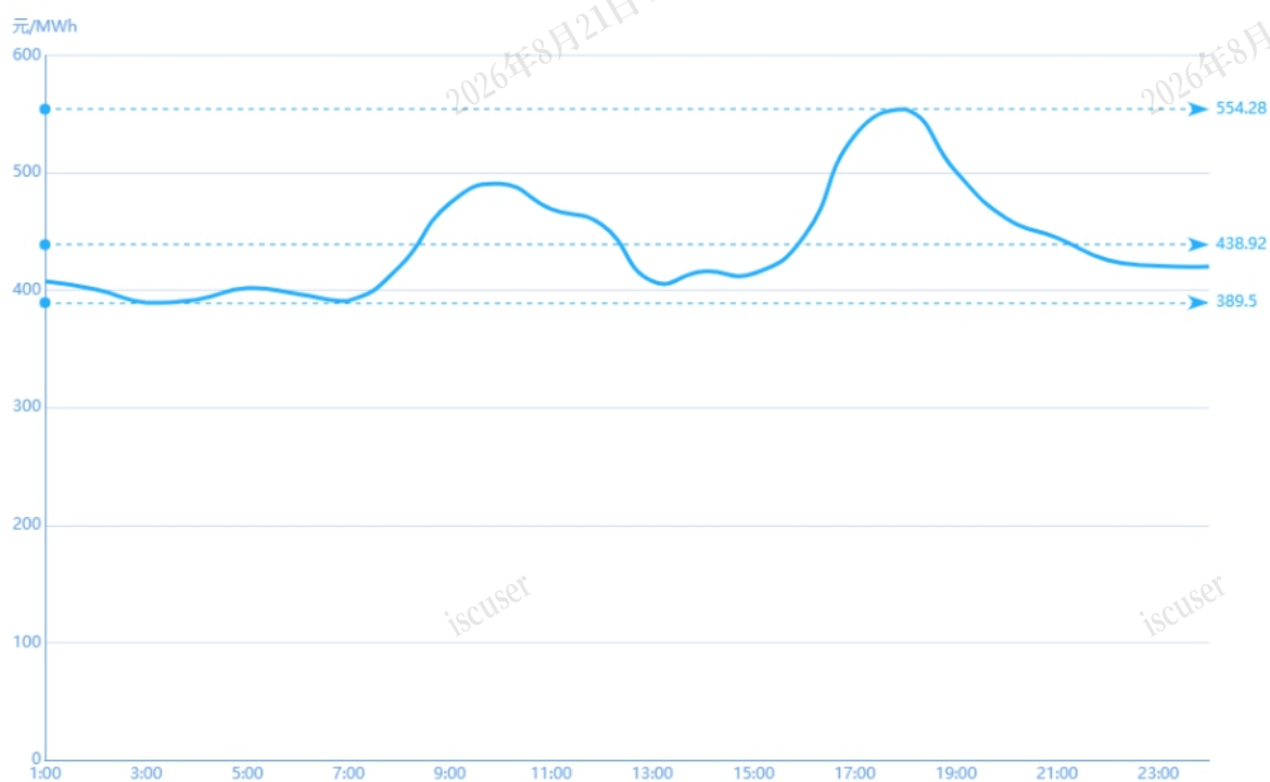
图3 12月26日实时市场用电侧价格
