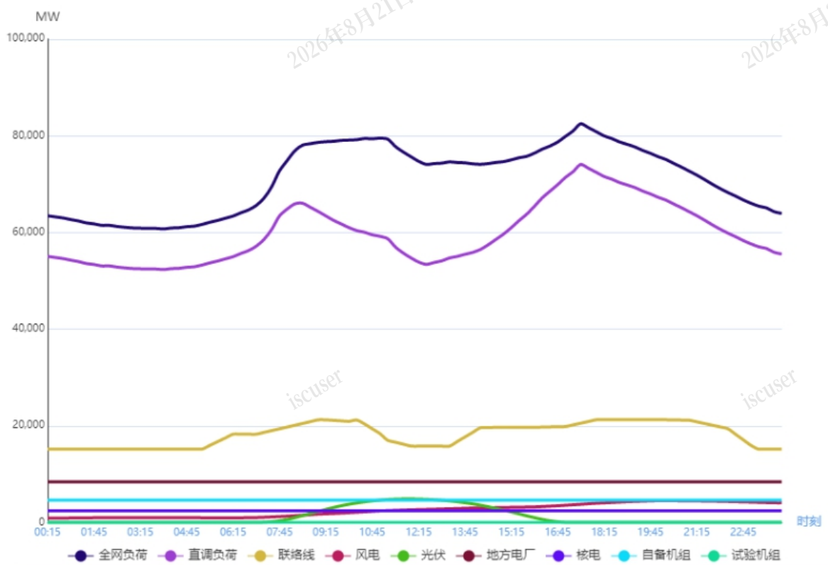
图 1 12 月 27 日负荷及电源出力预测情况
