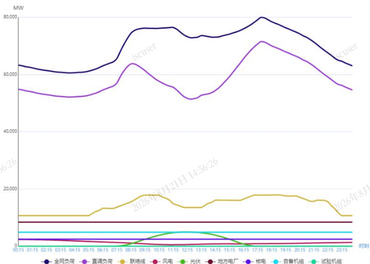
图1 1月2日负荷及电源出力预测情况
