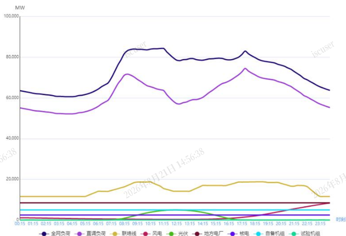
图1 1月5日负荷及电源出力预测情况
