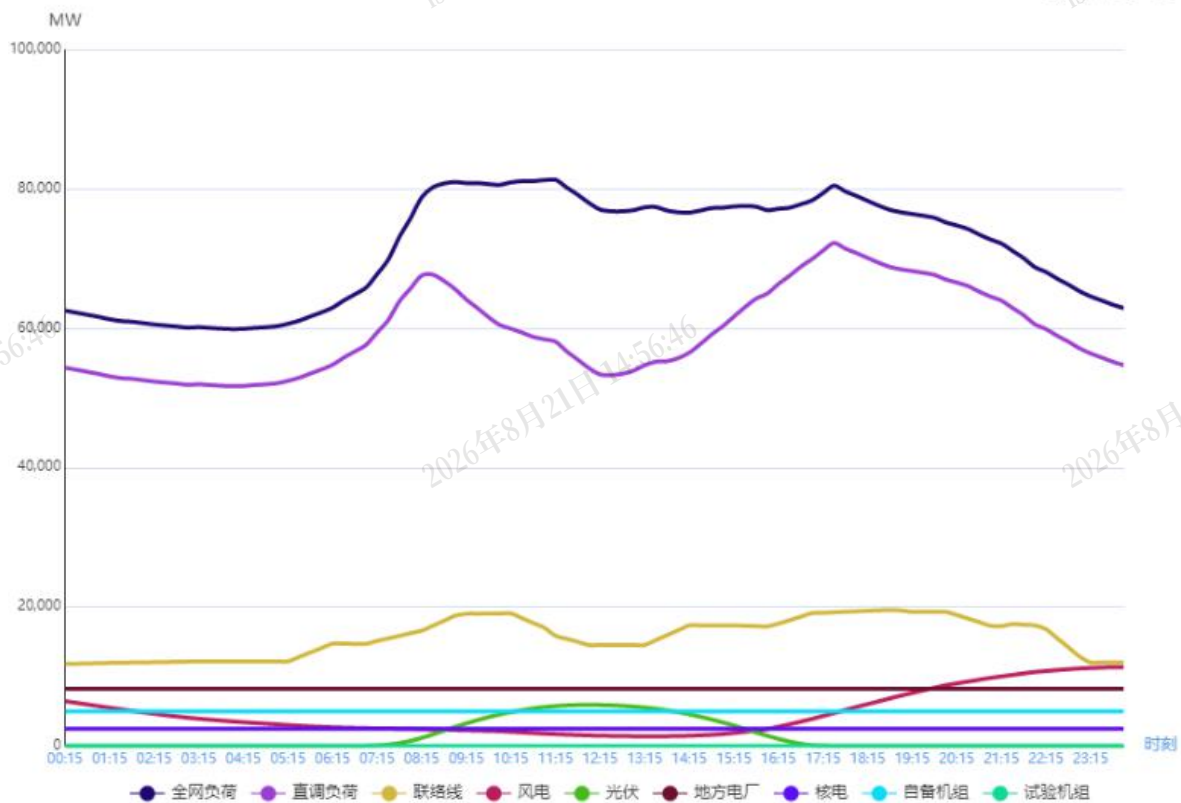
图1 1月7日负荷及电源出力预测情况
