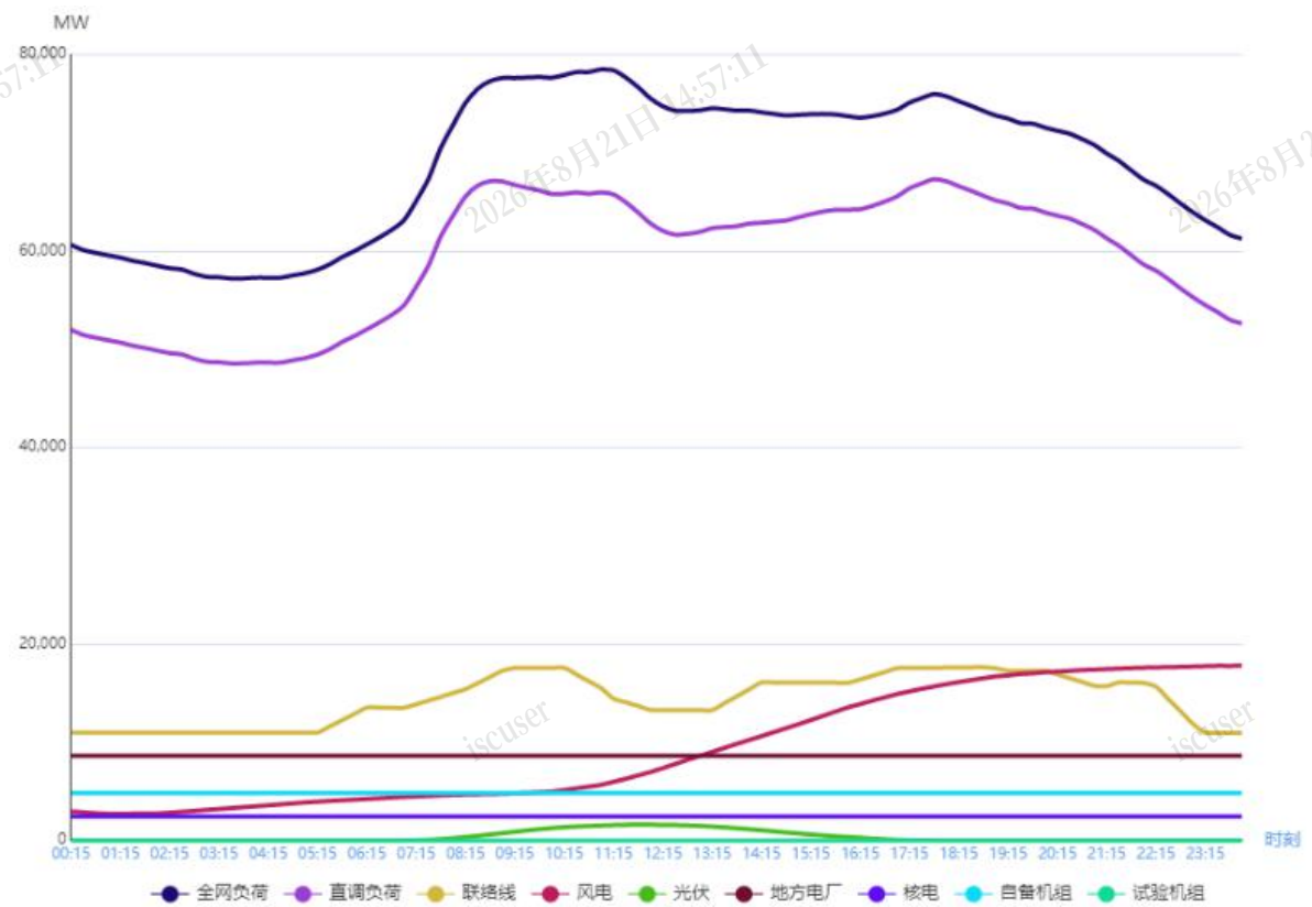
图 1 1月13日负荷及电源出力预测情况
